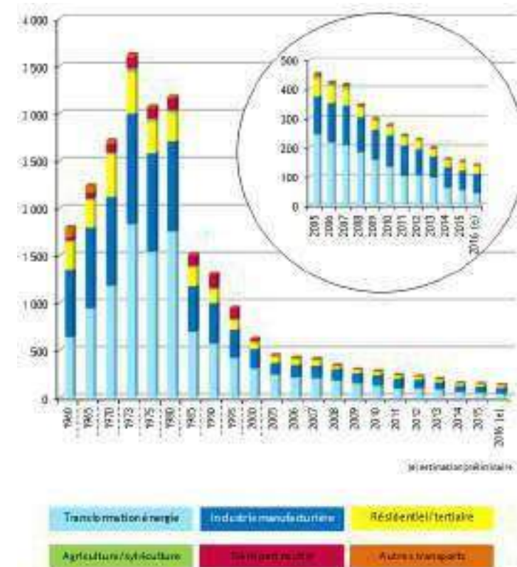
Emissions atmosphériques de SO2 par secteur en France métropolitaine en kt
